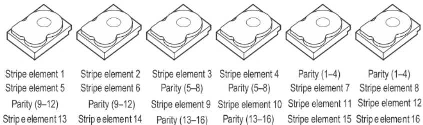
Figure 9. Exemple de parité distribuée double (RAID 6)
